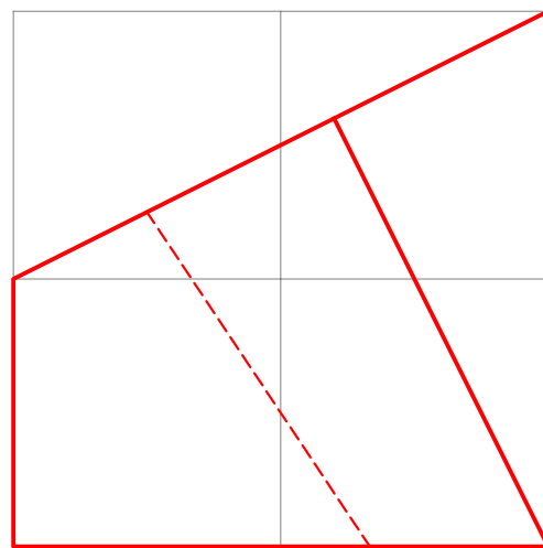
Kreuzriss (A.v.I.) A'''
