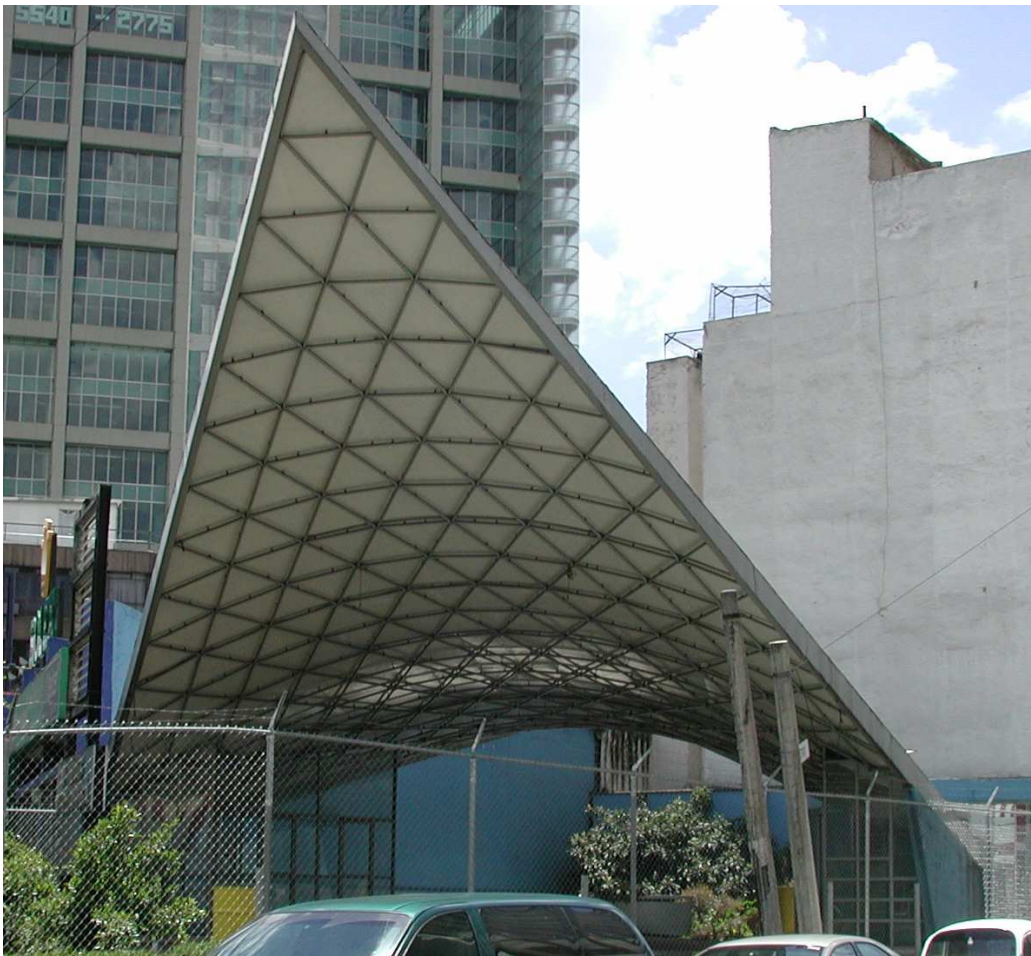
Abbildung 6: Hyperbolisches Paraboloid
