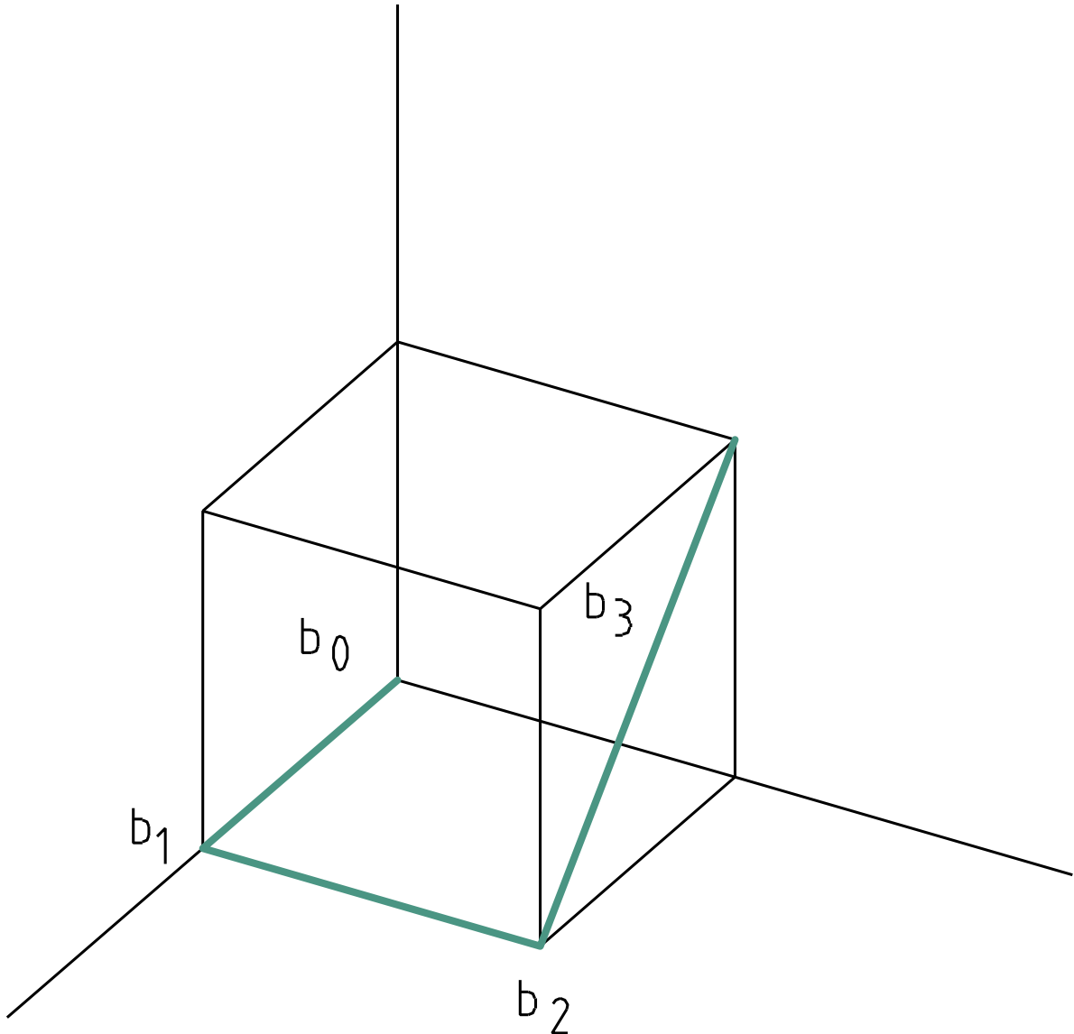
Abbildung 2: Konstruktion einer Bezierkurve
